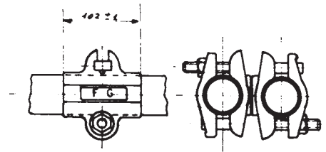
GIUNTO GIREVOLE
