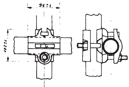
GIUNTO ORTOGONALE
